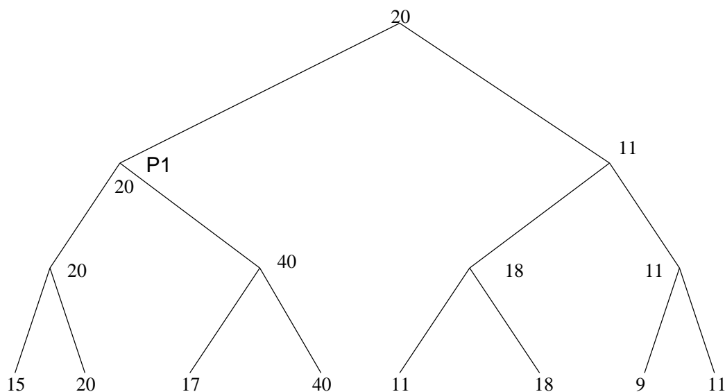
Figure 15.5 – Exemple d’arbre minimax
